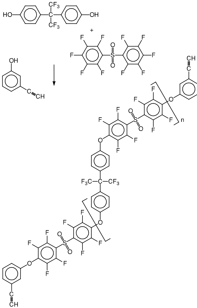
الشكل (7-12): اصطناع بوليميرات PAES المفلورة المنتهية بالإيثينيل 105,104
